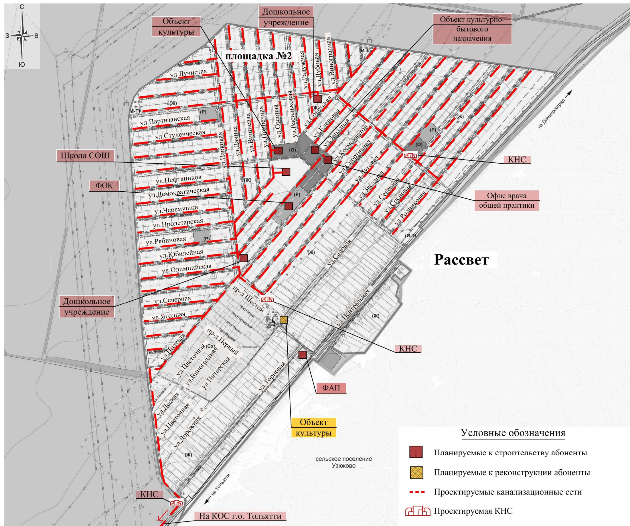
Рисунок 3.4.6.1- Расположение перспективных объектов системы водоотведения на перспективной площадке №2 п. Рассвет
