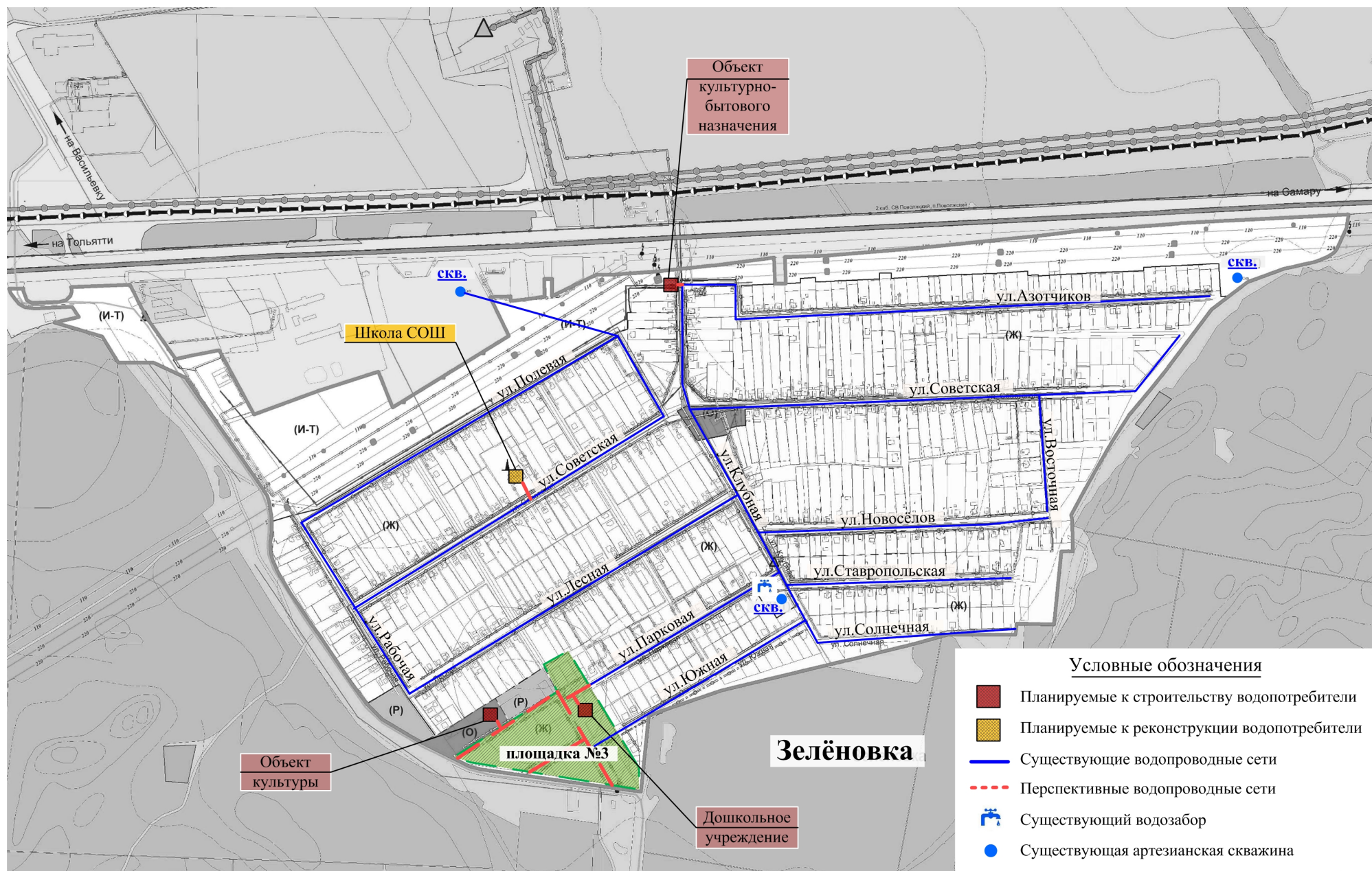
Рисунок 2.4.9.2 - План развития централизованных систем водоснабжения села Зелёновка
